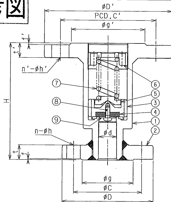
入口フランジ：RF の場合
