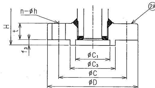
入口フランジ：ミゾ形 凸 の場合
