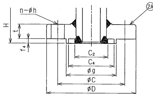
入口フランジ：ミゾ形 凹 の場合
