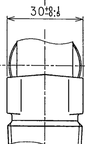
スパナ掛部の寸法
