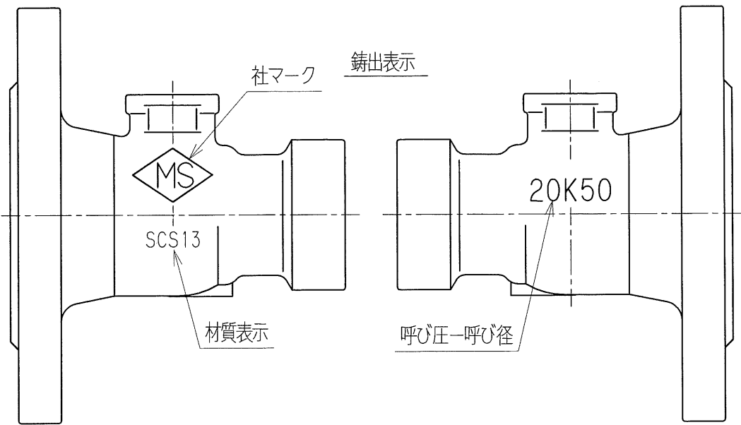
刻印表示例 (ボディフランジ側面)
