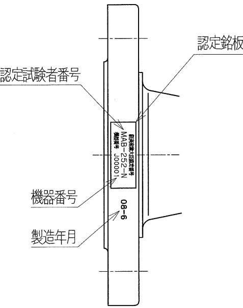
刻印表示例 (ボディフランジ側面)
