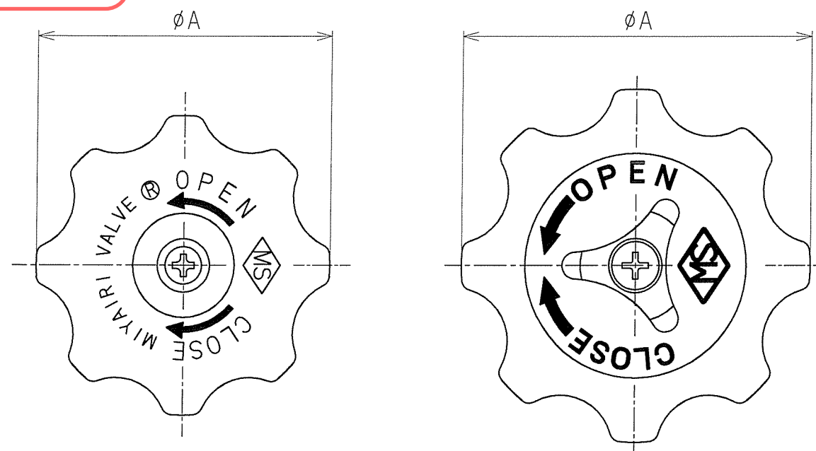
LPI-8のハンドル形状
