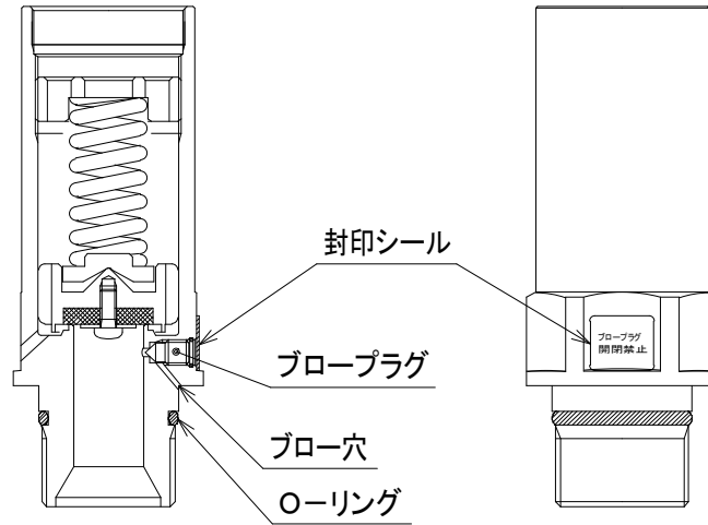
図1 LPR-680Jの構造
