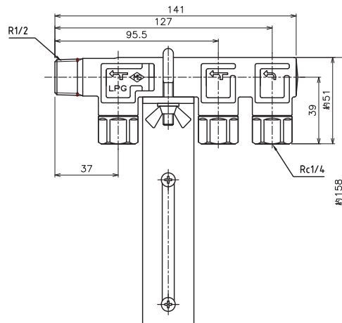
簡易ヘッダー6本立て MH-15CN-12 (R1/2)
