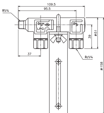
簡易ヘッダー4本立て MH-8CN-09 (R1/4)
