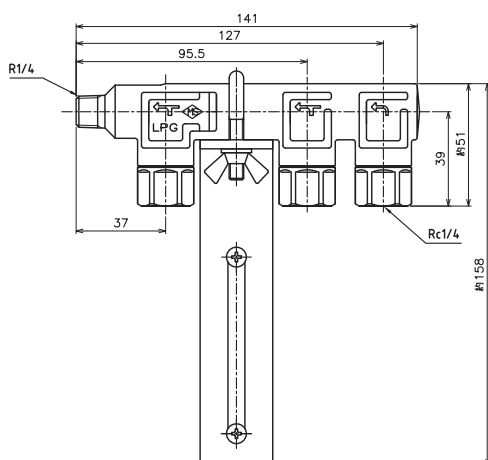
簡易ヘッダー6本立て MH-8CN-11 (R1/4)
