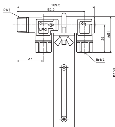
簡易ヘッダー4本立て MH-15CN-10 (R1/2)
